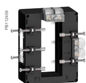
METSECT5DHxxx
