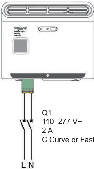
HeatTag sensor DIN mounted
