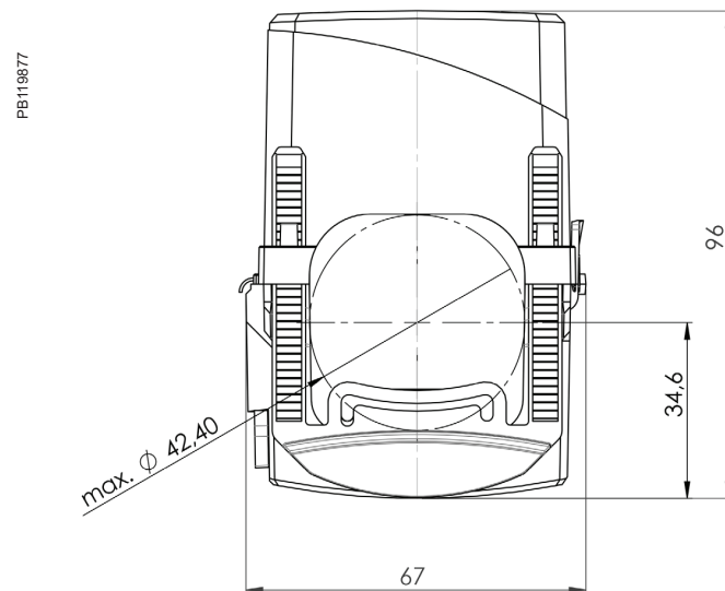
HJ Dimensions
