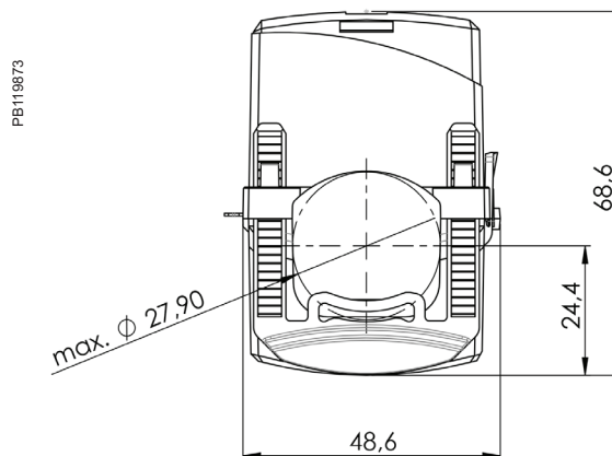
HD Dimensions
