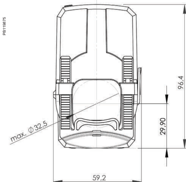
HG Dimensions
